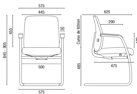
40.106 SI / 40.206 SI Aproximação
