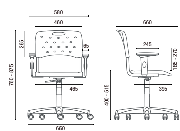
35004 Giratória Base em Aço com Capa
