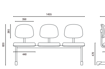
4009 Secretária Longarina Larguras sem Braço: 2L - 950mm 3L - 1455mm 4L - 1965mm 5L - 2470mm
