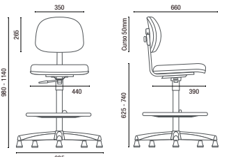
4022 BG Secretária Stool
