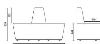
36.818 Módulo Ponta Encosto Interno 180°
