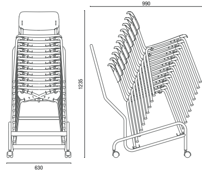
Carrinho Joy Empilhamento máximo: 10 unidades
