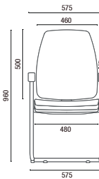
38006 SI Aproximação Alta com Braços Integrados
