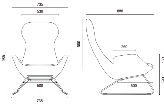
36.111 Poltrona Fixa - Base Frame
