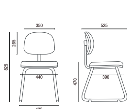
4008 A Secretária Aproximação
