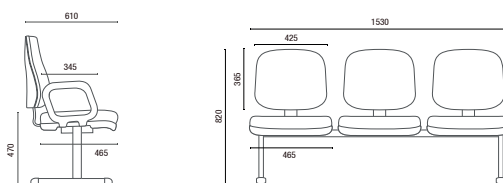
4110 Executiva Longarina Larguras sem Braço: 2L - 995mm 3L - 1530mm 4L - 2065mm 5L - 2595mm
