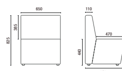
36.865 Módulo Reto 650mm
