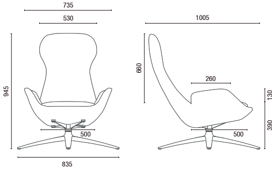
36.101 Poltrona Giratória - Base em Alumínio Polido
